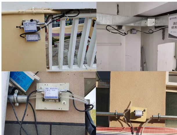
陕西延安某 危房 沉降监测
