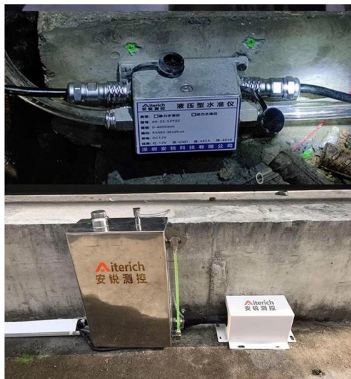
江西瑞金某 危房 监测
